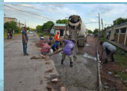
Proyecto de pavimentación con concreto hidráulico en la Col Buena Vista
